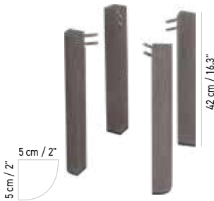
JEU DE 4 PIEDS POUR TABLE BASSE SET OF 4 FEET FOR LOW TABLE
